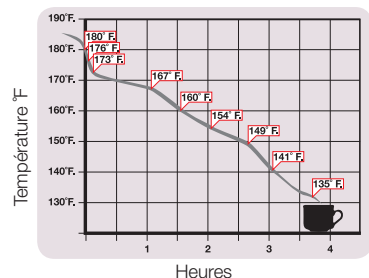
Test de rétention de chaleur SwirlServe®
